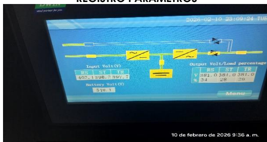
TENSION DE BATERIAS DEL UPS
